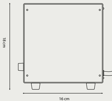
Bočný pohľad
